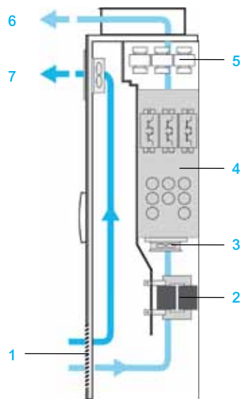
IP 23机柜
